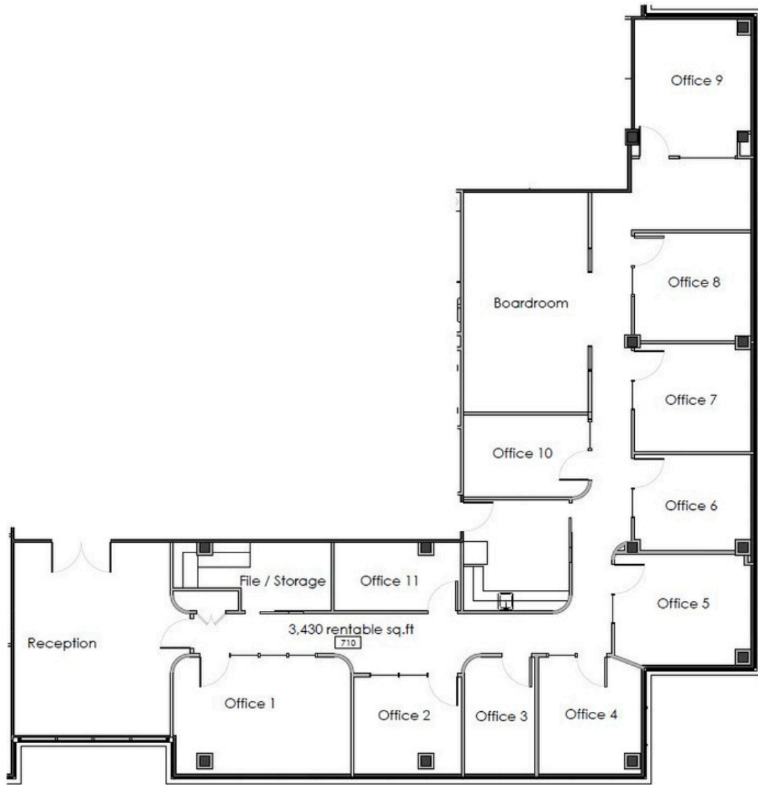
#710 - TENANT PLAN SCALE - 1/4" = 1'-0"
